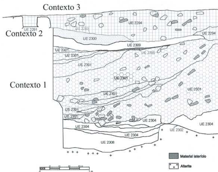
Figura 4 - Perfil estratigráfico "Este" del sondeo n° 8 de "As Cavalariças".
